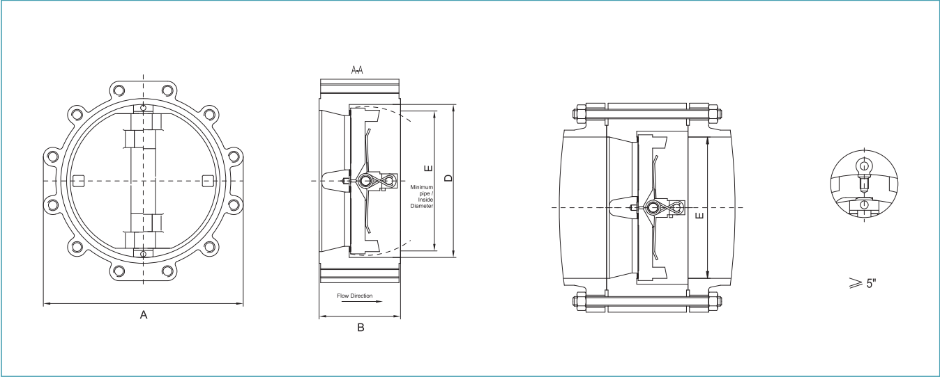
Lug type
